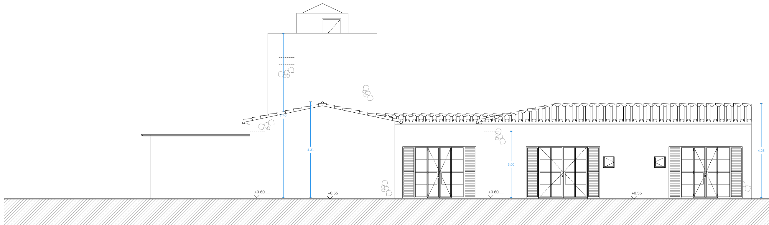
ALZADO LATERAL
