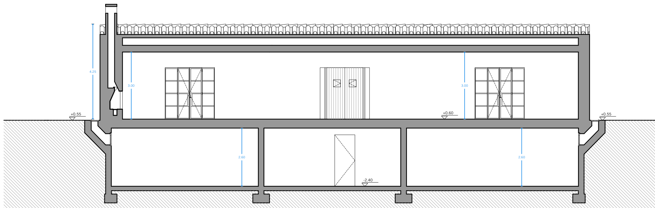
SECCIÓN LONGITUDINAL
