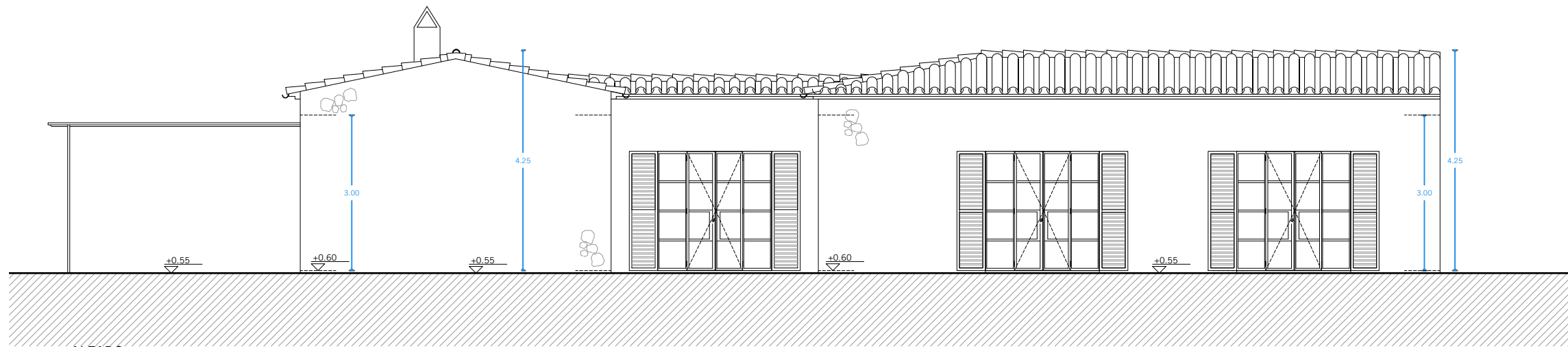
ALZADO LATERAL
